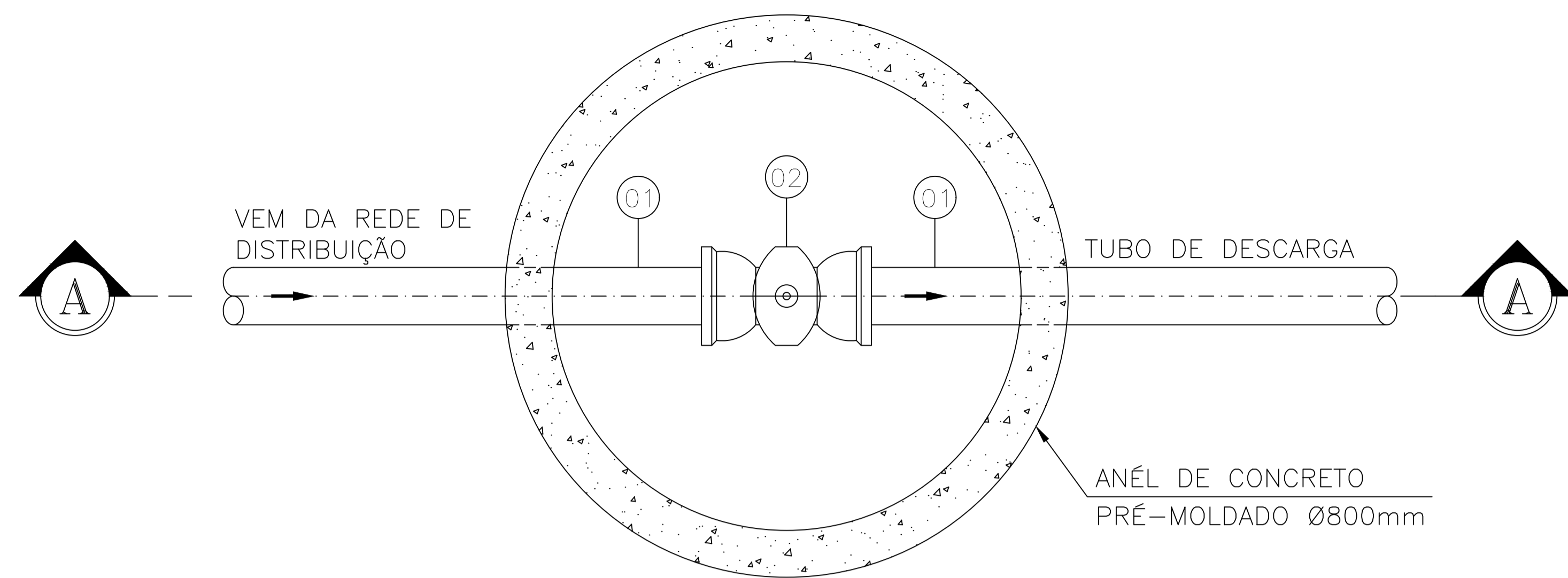
1 PLANTA BAIXA ESCALA 1:15
