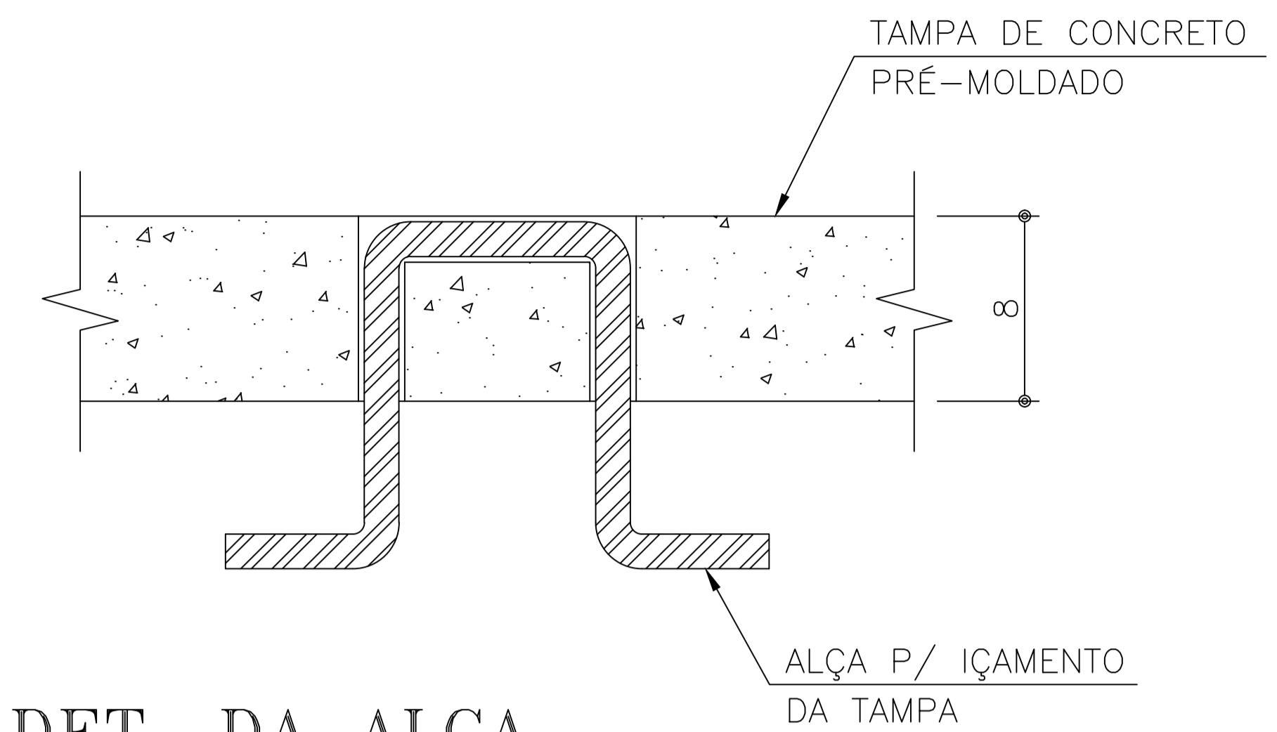
4 DET. DA ALÇA ESCALA 1:5
